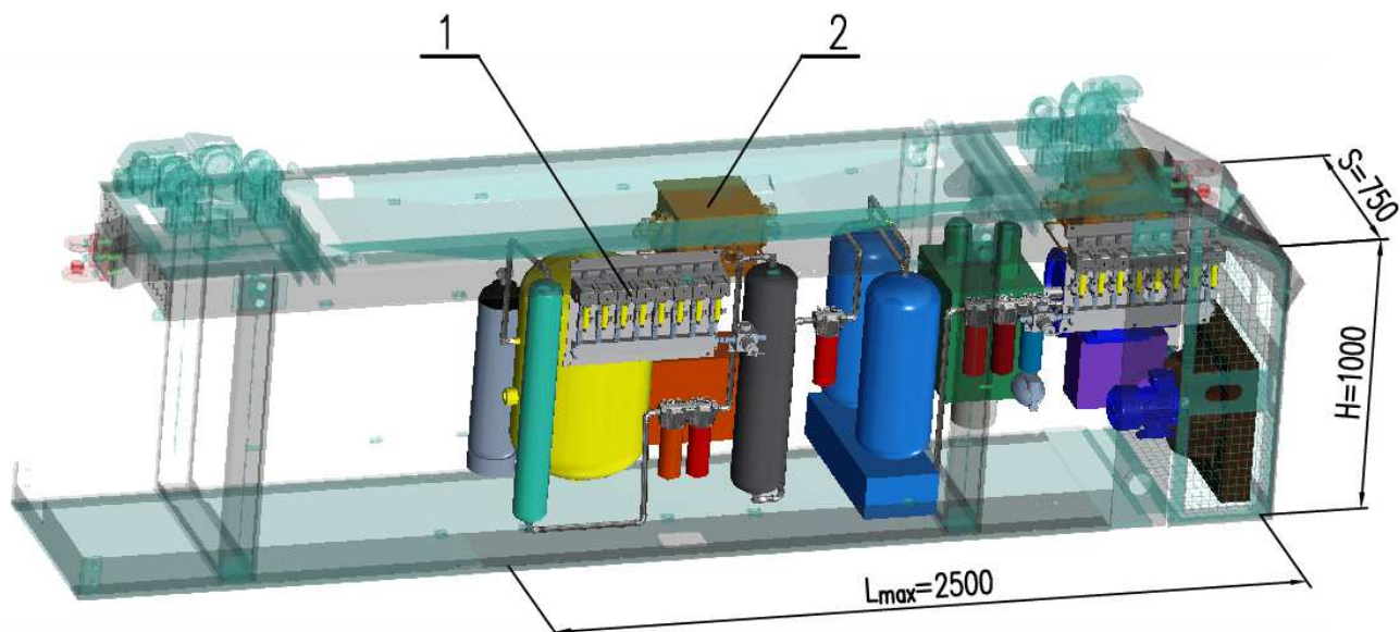
Rys.1 Przykładowy sposób zabudowy agregatu azotu w ramie (1 – układ inertyzacji, 2 – skrzynka ognioszczelna)
