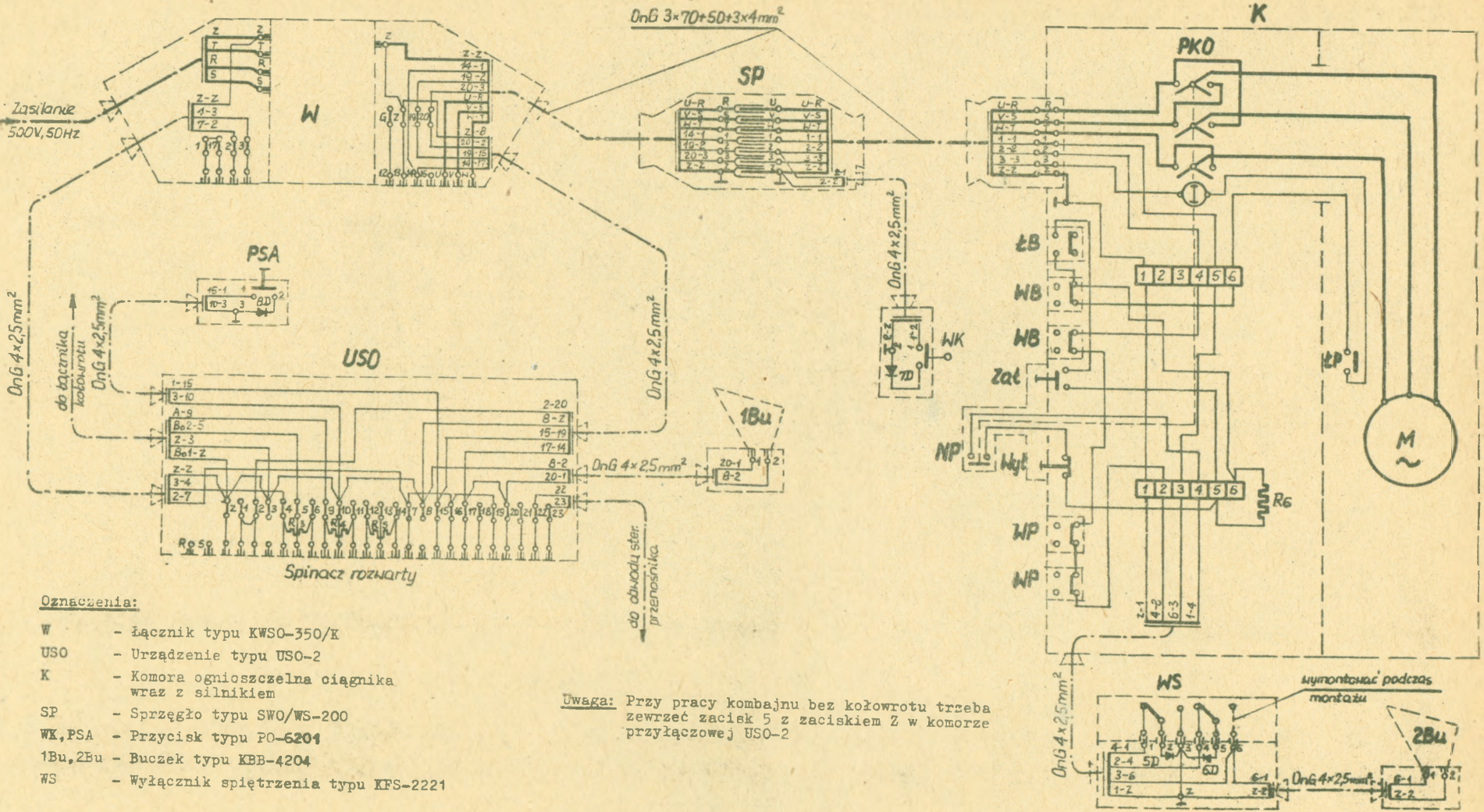
Rys. 12. Montażowy potaczeń kombajnu KB-125.
