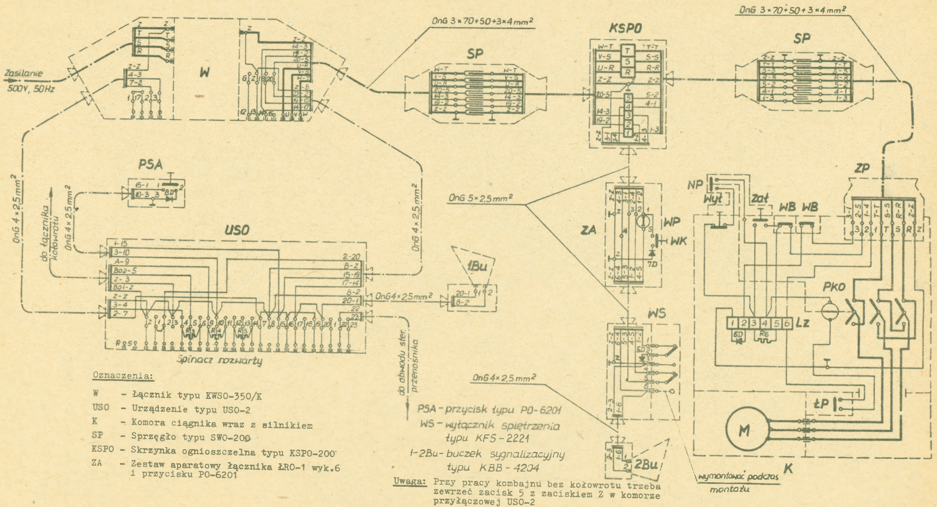
Rys. 10 Montażowy układ połączeń kombajnu KWB-3
